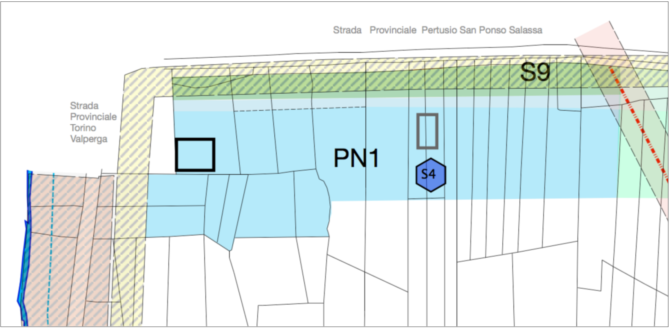
estratto PRGC - comune di San Ponso area PN1 - area produttiva nuovo impianto scala 1:2000
